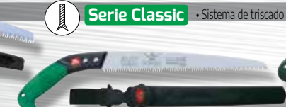
Serrucho recto con funda JS 240 240 mm. (Cod: 08230605) JS 300 LH 300 mm. (Cod: 08230610) JS 270 LH 270 mm. (Cod: 08230607)
